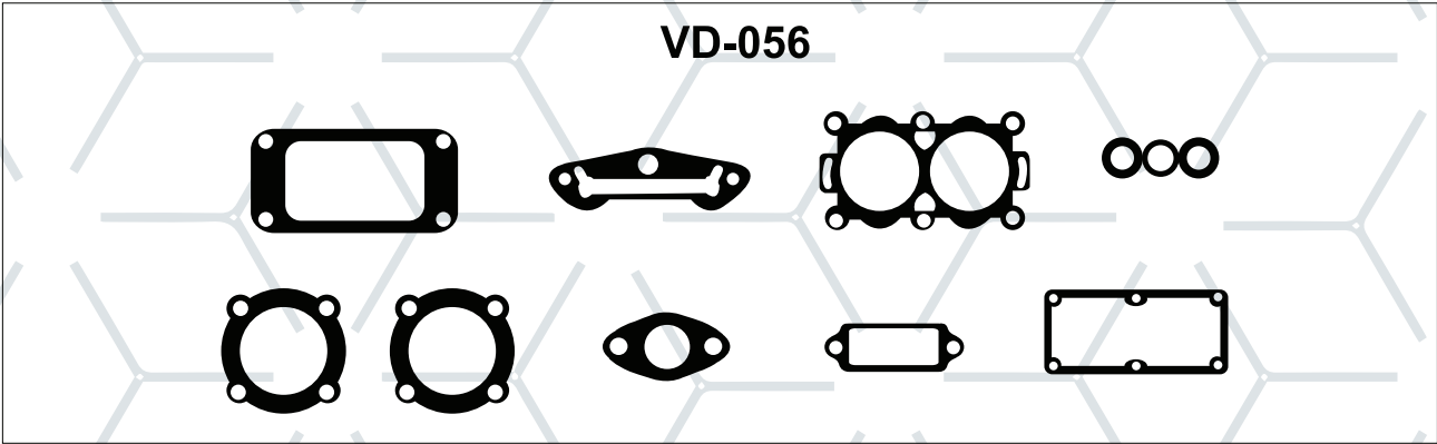
JUEGO DE JUNTAS PARA COMPRESOR MIDLAND TIPO EL-1300 / RNT26, EL13020 2" 3/4
